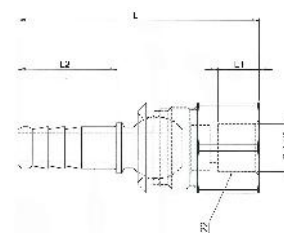
Schlauchtülle, Innengewinde
