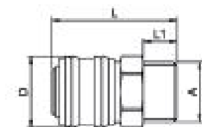
Außengewinde
