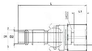
Nippel, drehbar
