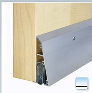
Planet Sockel mit Planet FT Profil 13 x 30 mm
