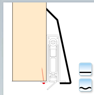
Option: Planet Sockel für Planet GH 14 x 47,5 mm (auf Anfrage)
