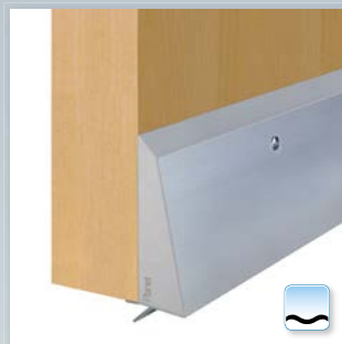
Planet Sockel mit Abdeckplatte und Planet RF Profil 13 x 30 mm, Schrägrippe
